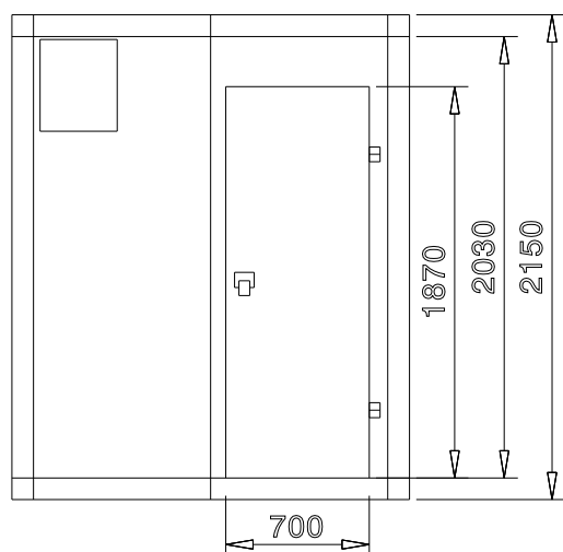
Zij aanzicht
